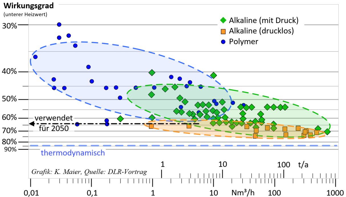
Abb. 5-1 Wirkungsgrade bestehender Anlagen
