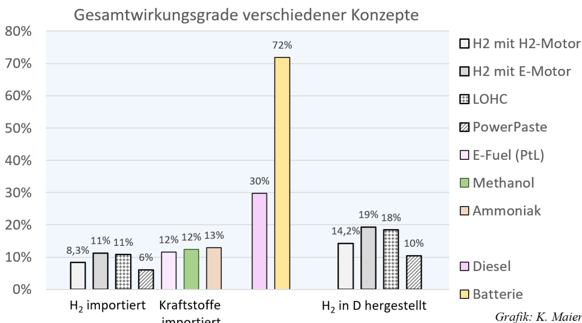
Abb. 6-2 Wirkungsgrade Mobilität
