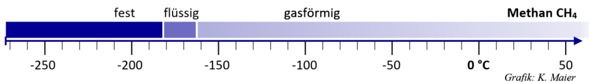
Abbildung 5-1 Aggregatzustände Methan bei Normaldruck
