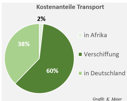
Abb. 7-4 Kostenanteile am Transport
