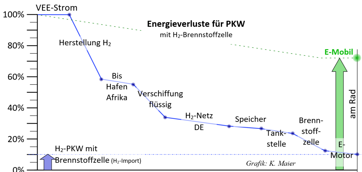
Abb. 6-3 Energieverlusttreppe PKW
