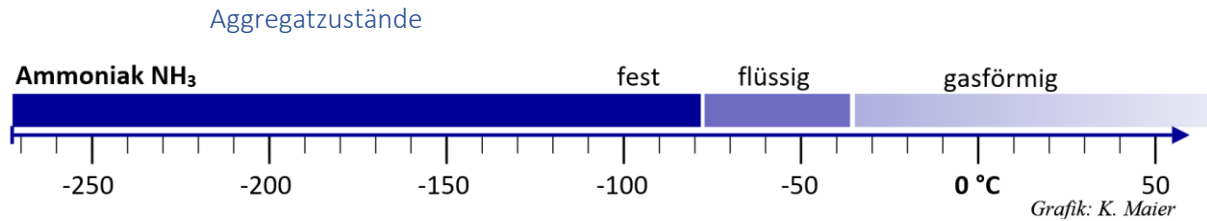
Abbildung 5-2 Aggregatzustände Ammoniak bei Normaldruck
