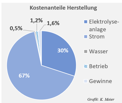
Abb. 7-3 Kostenanteile an H 2 -Herstellung
