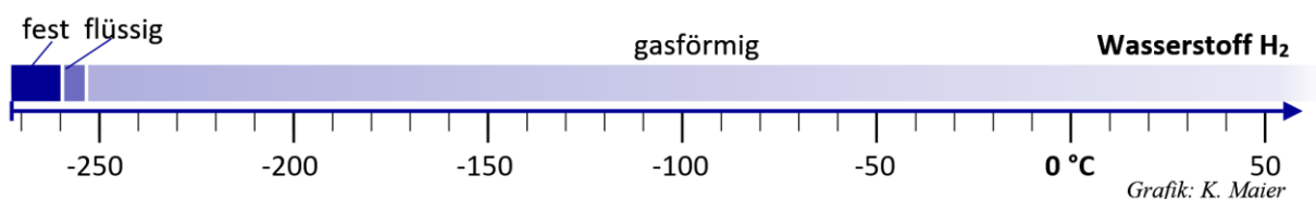
Abb. 5-2 Aggregatzustände Wasserstoff bei Normaldruck
